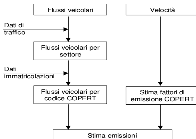
Figura 2-2 – Schema metodologico
